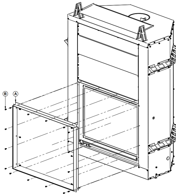
Figure 28.2 Contour pour finition de maçonnerie
