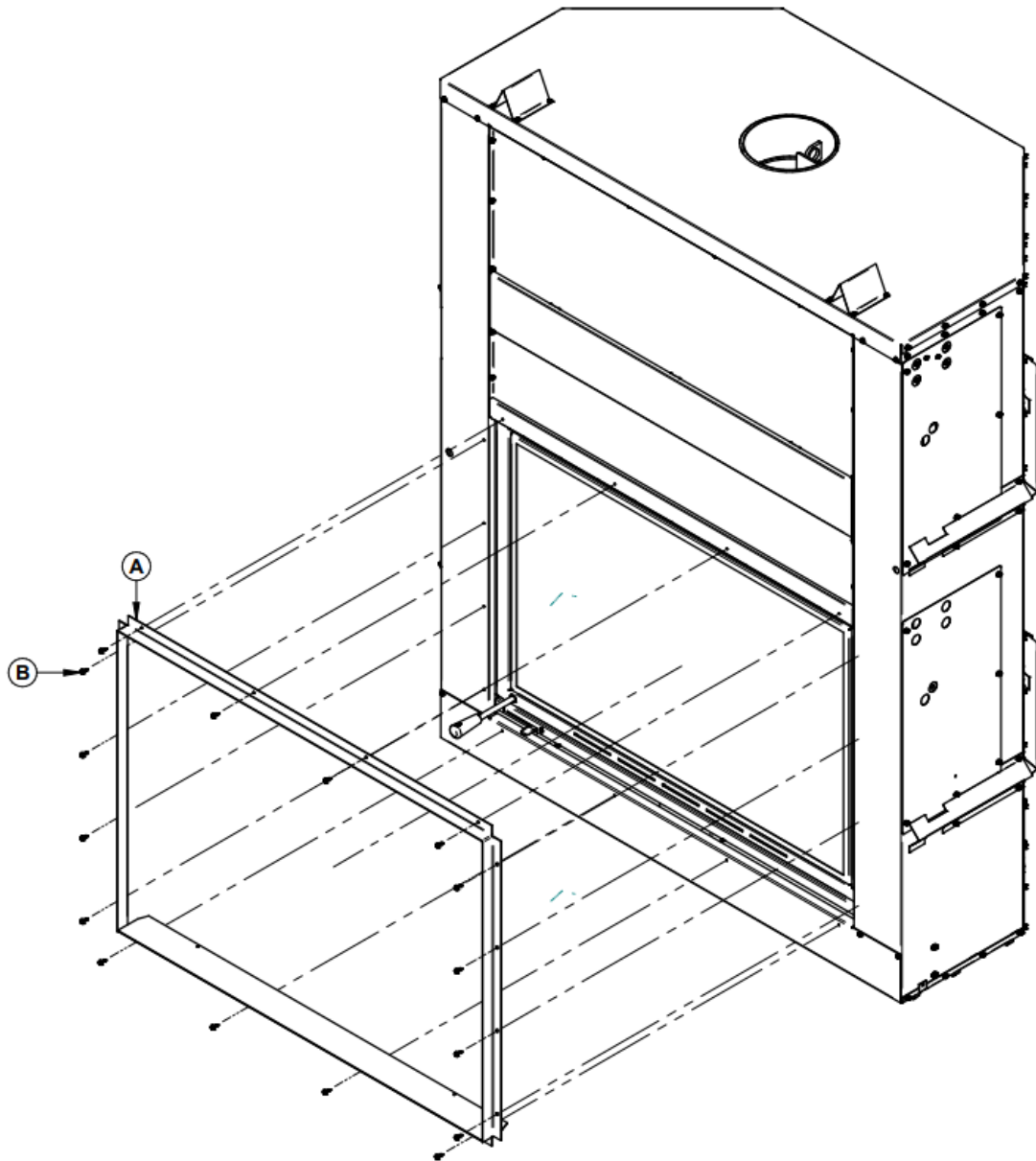
Figure 25 Contour pour finition de maçonnerie
